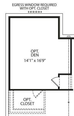
Optional Den
